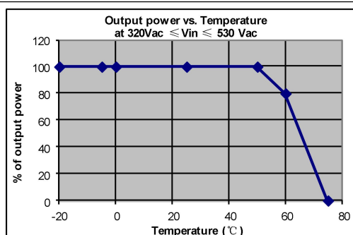
图 1.2 DR750-10000 系列温度限功率曲线
