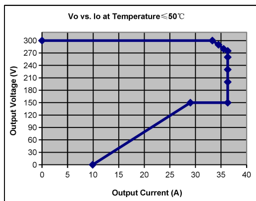
图 2.1 DR240-10000 输出 V-I 曲线
