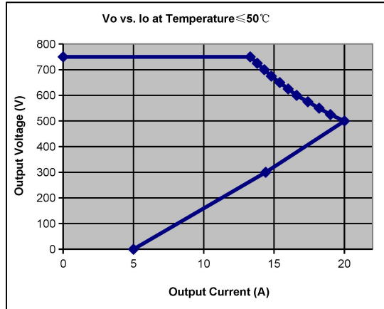
图 2.4 DR750-10000 输出 V-I 曲线
