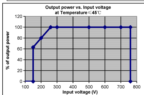
图 1.1 DR750-10000 系列输入限功率曲线
