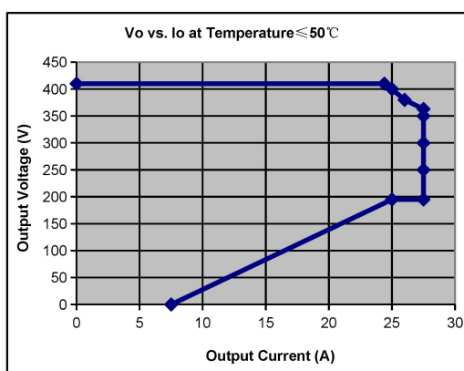
图 2.2 DR336-10000 输出 V-I 曲线
