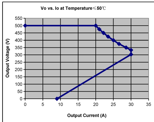
图 2.3 DR500-10000 输出 V-I 曲线
