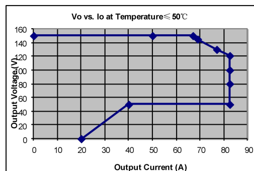
图 2.2 LM150-10000 输出 V-I 曲线
