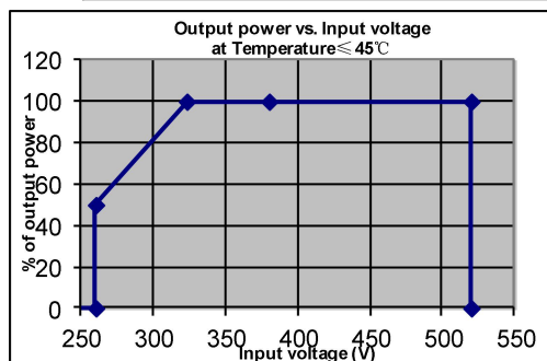
图 1.1 LM100-10000 系列输入限功率曲线
