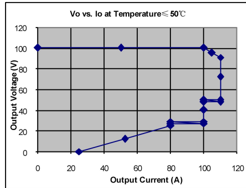
图 2.3 LM100-10000 输出 V-I 曲线
