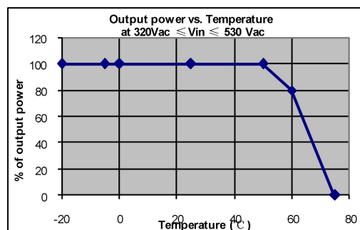
图 1.2 LM100-10000 系列温度限功率曲线
