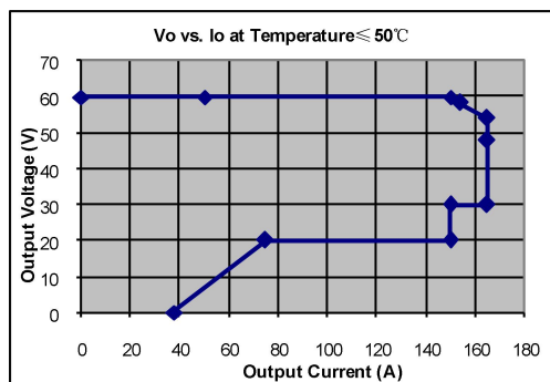
图 2.1 LM48-9000 输出 V-I 曲线
