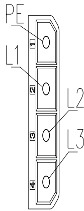
图 3: 输入插座定义图
