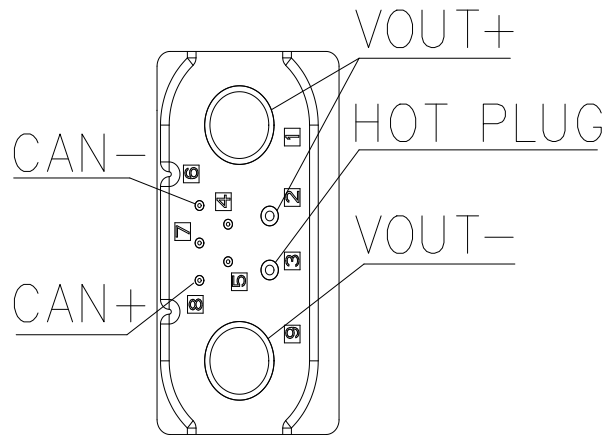
图 4: 输出插座定义图
